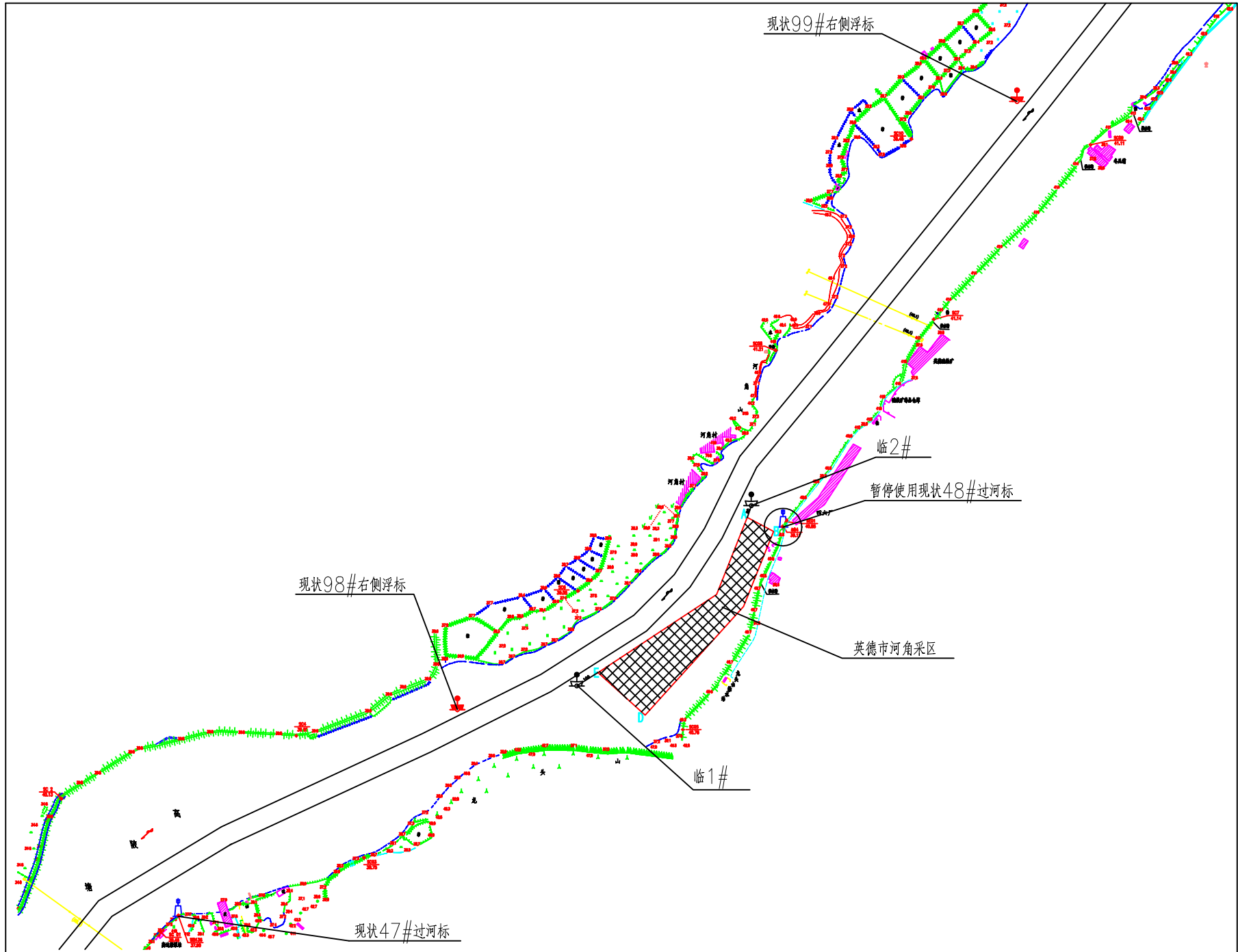
北江干流清远河段2020年度英德市河角可采区采砂工程施工项目航标配布示意图
