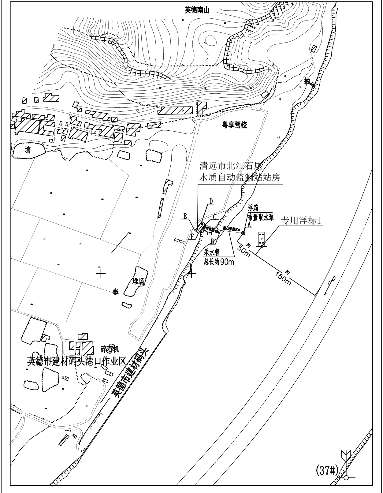
清远市北江石尾水质自动监测站航标配布示意图
